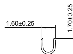
SEC:B-B
