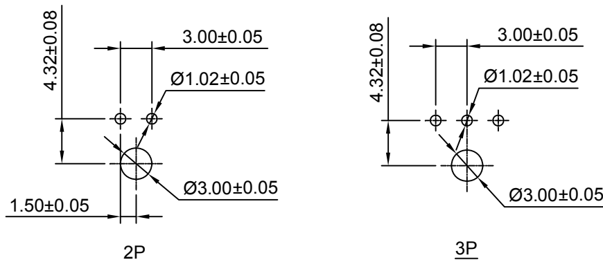
P.C.B LAYOUT
