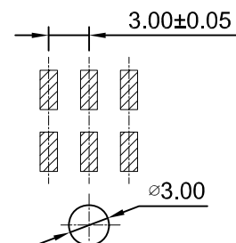
P.C.B LAYOUT (2x1P~2x3P)
