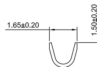
SEC:B-B
