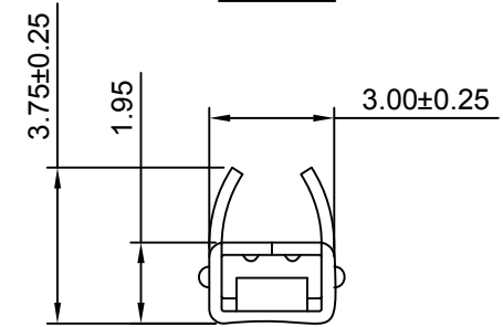
SEC:B-B
