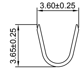
SEC:B-B
