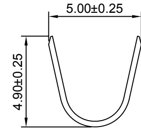
SEC:A-A
