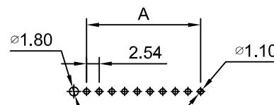
P.C.B LAYOUT Type 2
