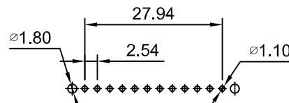
P.C.B LAYOUT Type 3
