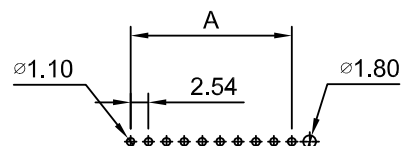
P.C.B LAYOUT Type 1
