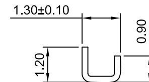
SEC:A-A
