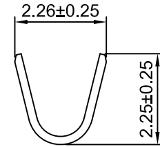
SEC:A-A
