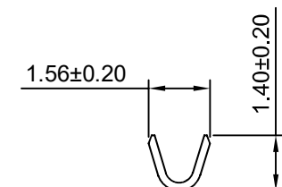
SEC:B-B
